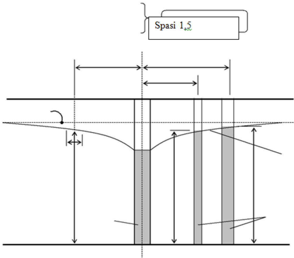
Gambar 1.2 Uji Pemompaan dari Suatu Sumur Uji dalam Lapisan Tembus Airyang Didasari oleh Lapisan Kedap Air (Asdak, 2000)
